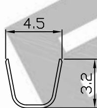
SEC A-A
